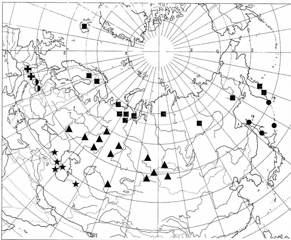
Map. Distribution of the Palearctic species of the Agyneta similis -group: ■ — A. similis ; ● — A. insulana ; ▲ — A. saaristoii ; ★ — A. mesasiatica ; ⊕ — A. milleri ; ⊕ — A. resslis & A. alpica . Карта. Распространение палеарктических видов группы Agyneta similis : ■ — A. similis ; ● — A. insulana ; ▲ — A. saaristoii ; ★ — A. mesasiatica ; ⊕ — A. milleri ; ⊕ — A. resslis & A. alpica .
